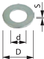
Washers (SRW) DIN 125
